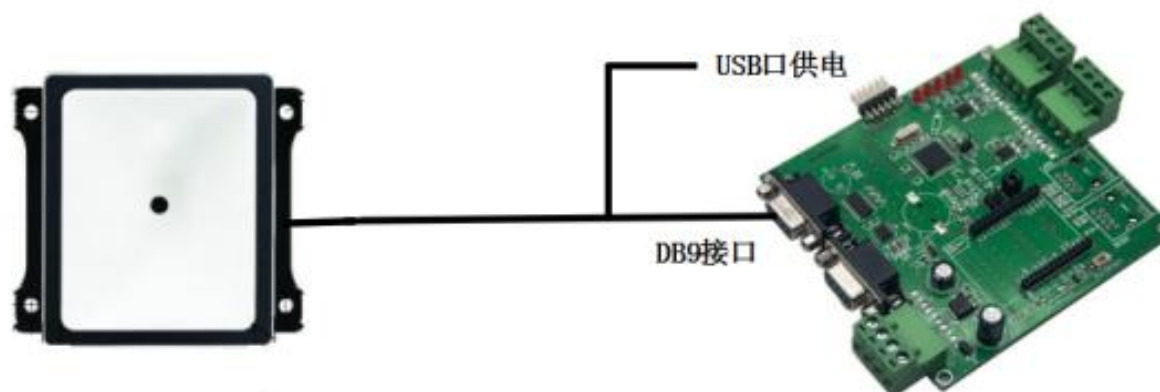
图 5.5 RS232 连接示意图
